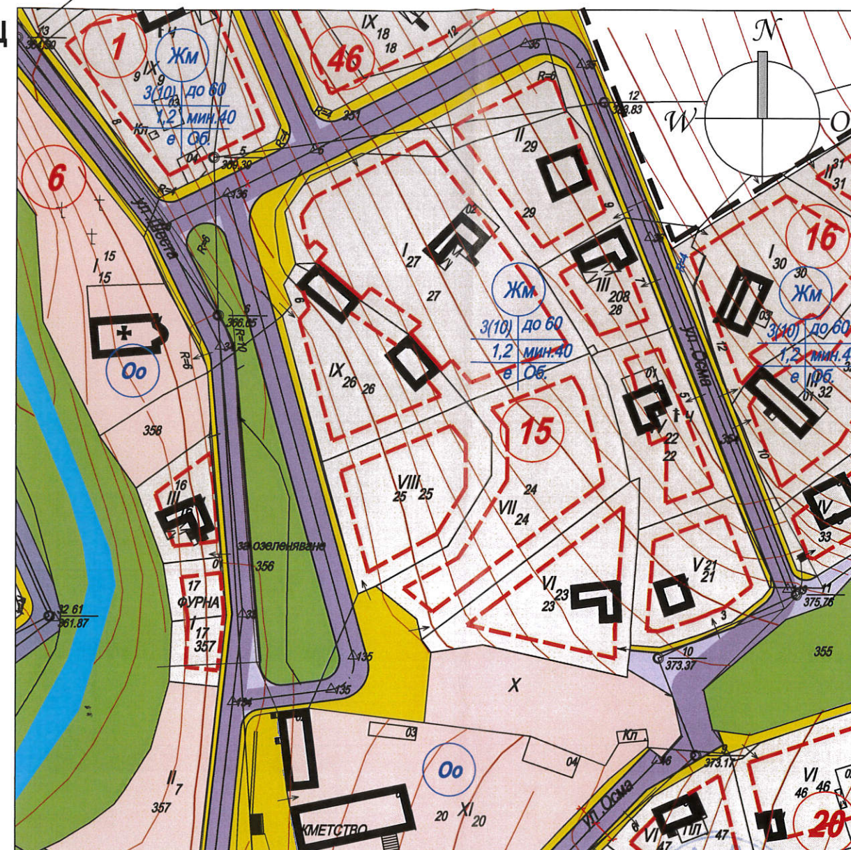
ЧАСТИЧНО ИЗМЕНЕНИЕ НА ПЛАНА ЗА ЗАСТРОЯВАНЕ М 1:1000
